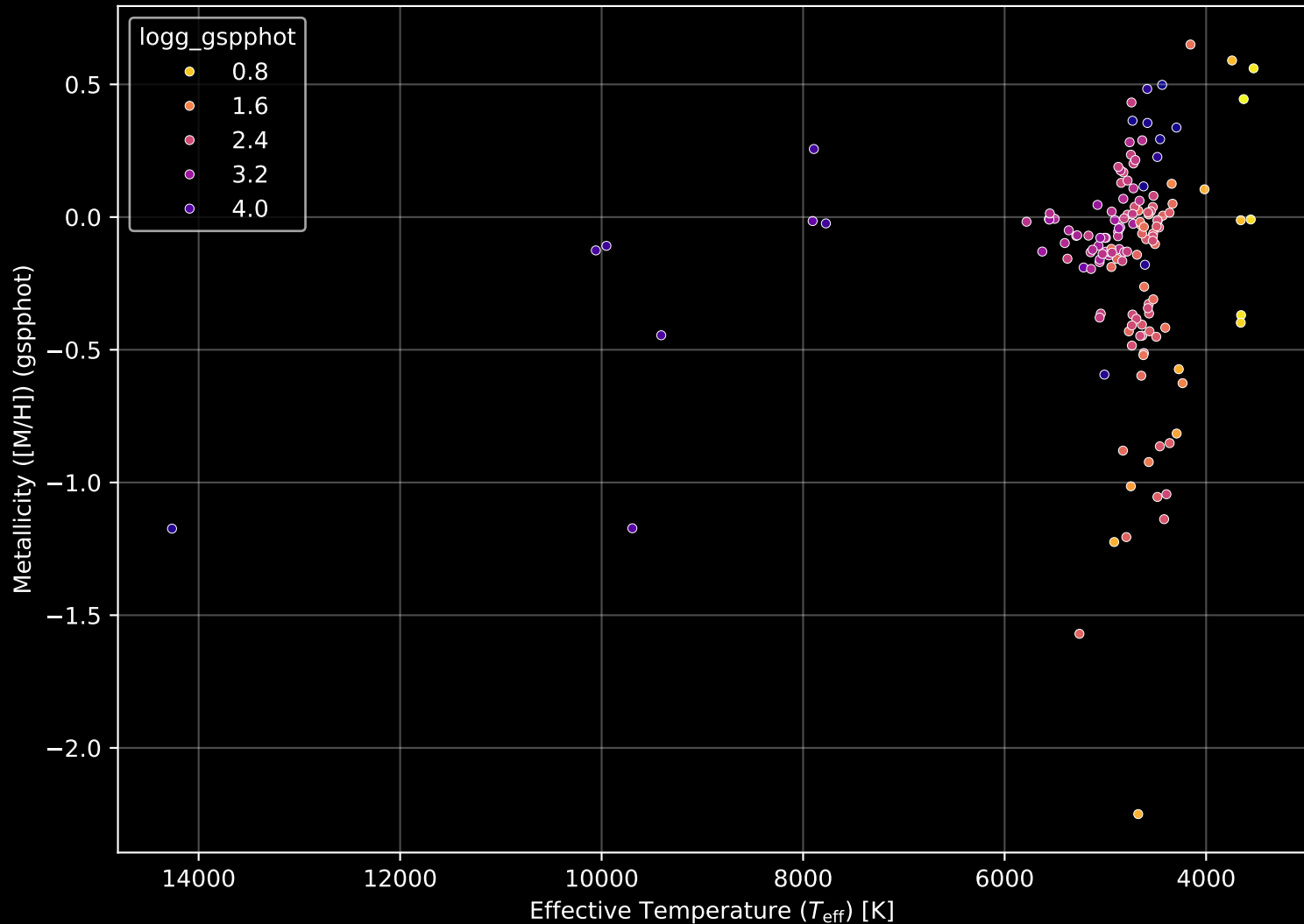
APOGEE DR17 Field: [020-14] Stellar Population Parameters (n= 148)
